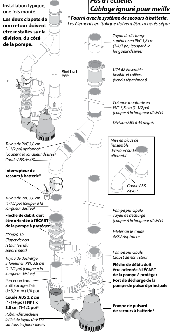
Fig 3 : Installation typique avec tuyau de décharge commun.
