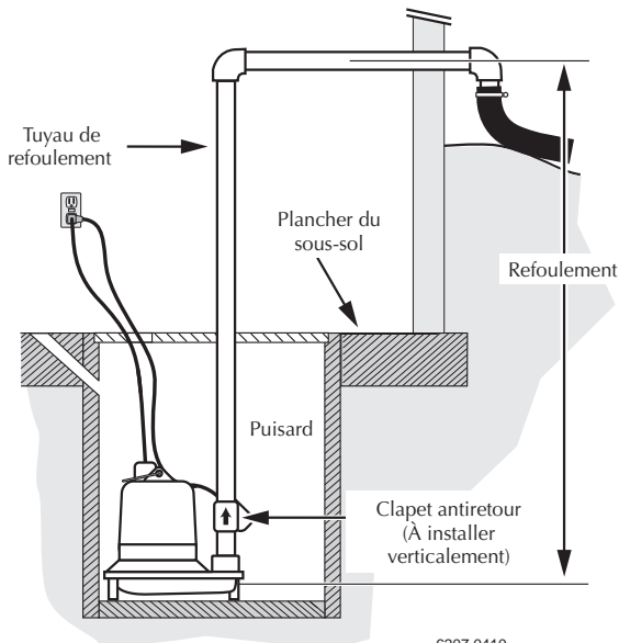
Figure 7 – REFOULEMENT : C'est la distance verticale à laquelle la pompe refoulera l'eau. Plus le refoulement est haut, moins la pompe débite.
